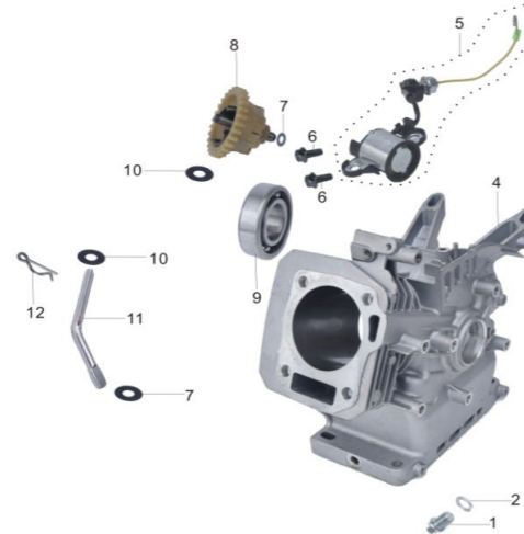
E-1 曲轴箱总成 CRANKCASE ASSY
